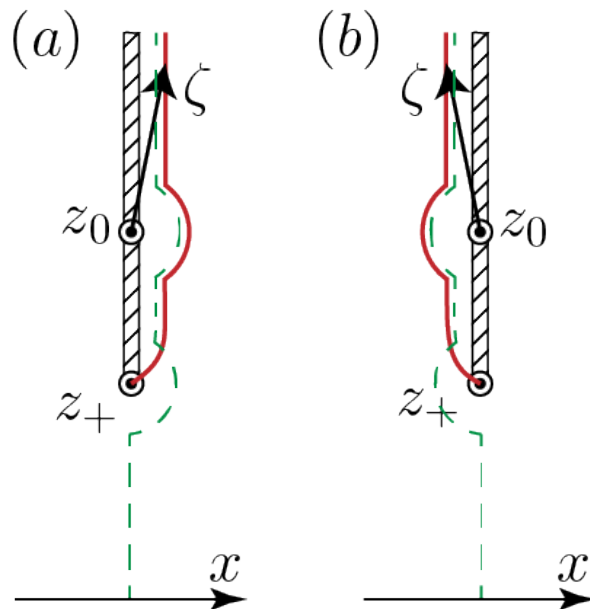
Рис. С.4: Контуры интегрирования (красные кривые) вдоль (а) правой антистоксовой линии, (b) левой антистоксовой линии. Зеленые пунктирные линии представляют путь, по которому следует аргумент p , когда точка \zeta перемещается от действительной оси, где p действительно и положительно, вверх вдоль правой (а) и левой (b) антистоксовых линий
