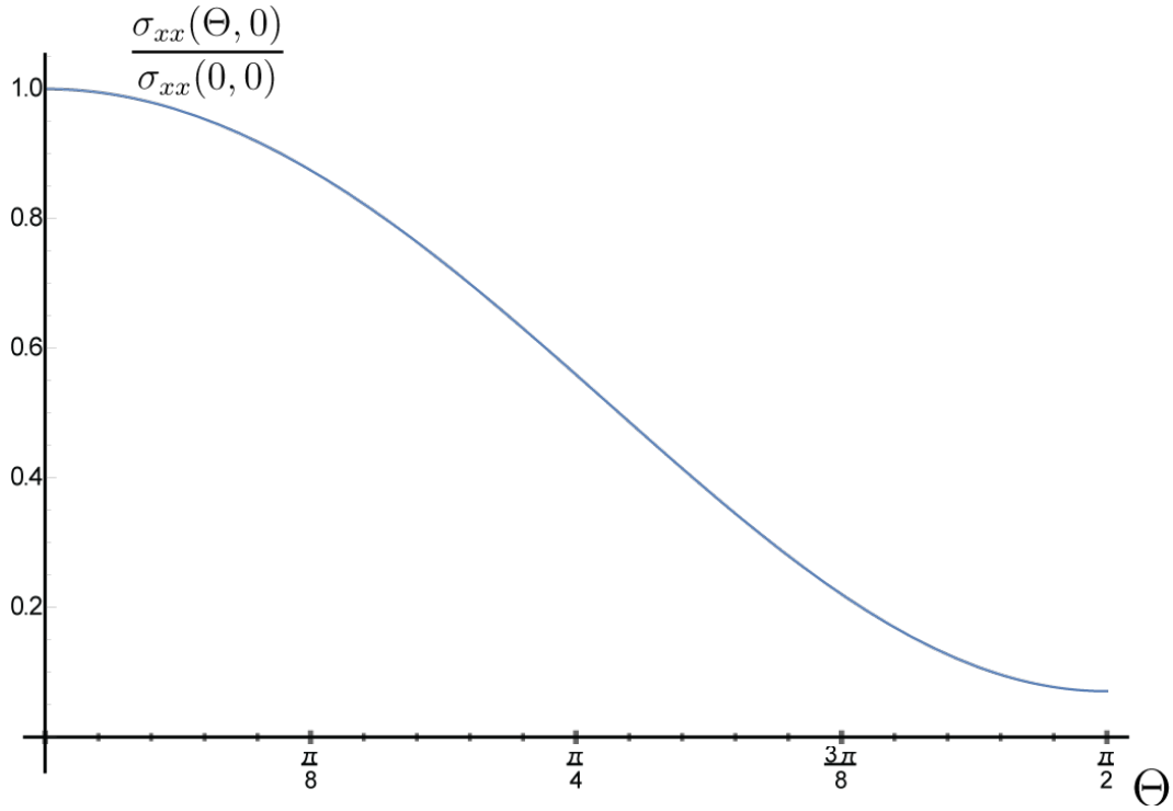
Рис. 2.5: Зависимость \Theta проводимости \sigma_{xx} при \Phi = 0 .
