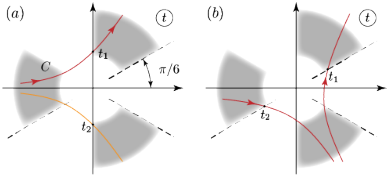
Рис. 3.3: (а) Расположение контура C , определяющего решение уравнения 3.25 для \arg s = 0 . Асимптотические серые области — это области, которые должны содержать конечные точки контура. (для сходимости интеграла). t_1, t_2 — это седла подынтегрального выражения. Контур, нарисованный с помощью точного пути наискорейшего спуска, проходящего через седло t_1 , оранжевая линия — это второй путь наискорейшего спуска, проходящий через седло t_2 . (б) Пути наискорейшего спуска и седла для \arg s = -2\pi/3
