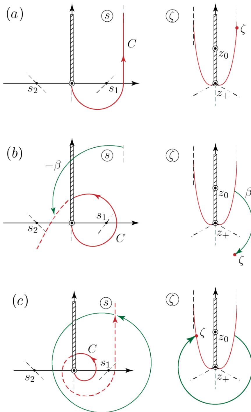
Рис. 3.5: (а) Справа: антистоксовы линии вблизи точки z_+ . Точка \zeta на правой антистоксовой линии такова, что волновая функция в этой точке представляет исходящую волну и должна соответствовать (3.53). Пунктирные линии — примерные направления антистоксовых линий. Слева: начальное расположение контура C для решения (3.56). s_1 и s_2 — седловые точки функции f(s, \zeta) в (3.57). Пунктирные линии — линии наискорейшего спуска f(s, \zeta) . (b) Справа: Аргумент \zeta находится на левой антистоксовой линии (повернут на 2\pi ). Слева: Контур C деформирован в спираль.
