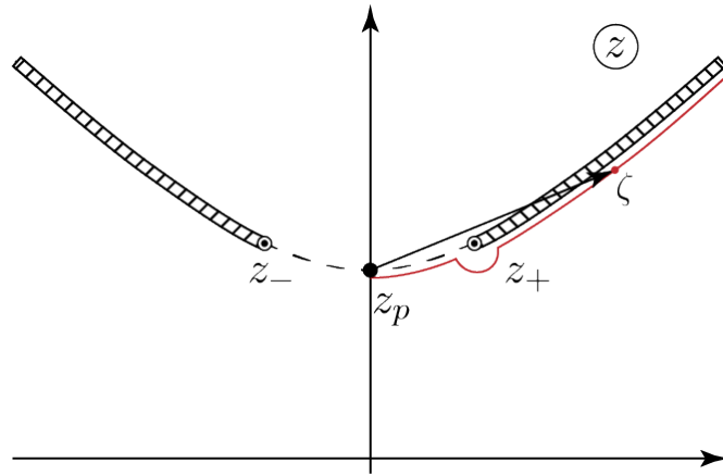
Рис. С.2: Кривые \text{Im}\varphi^2(z) = 0 для функции Лоренца \varphi(z) = (z^2 + 1)^{-1} . Кривые образуют гиперболу y = \sqrt{x^2 + 1} .
