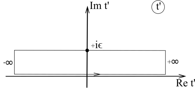
Рис. 1.2: Контур интегрирования в плоскости комплексного t' ; \epsilon — конечное положительное число, как и \pi - \epsilon .
