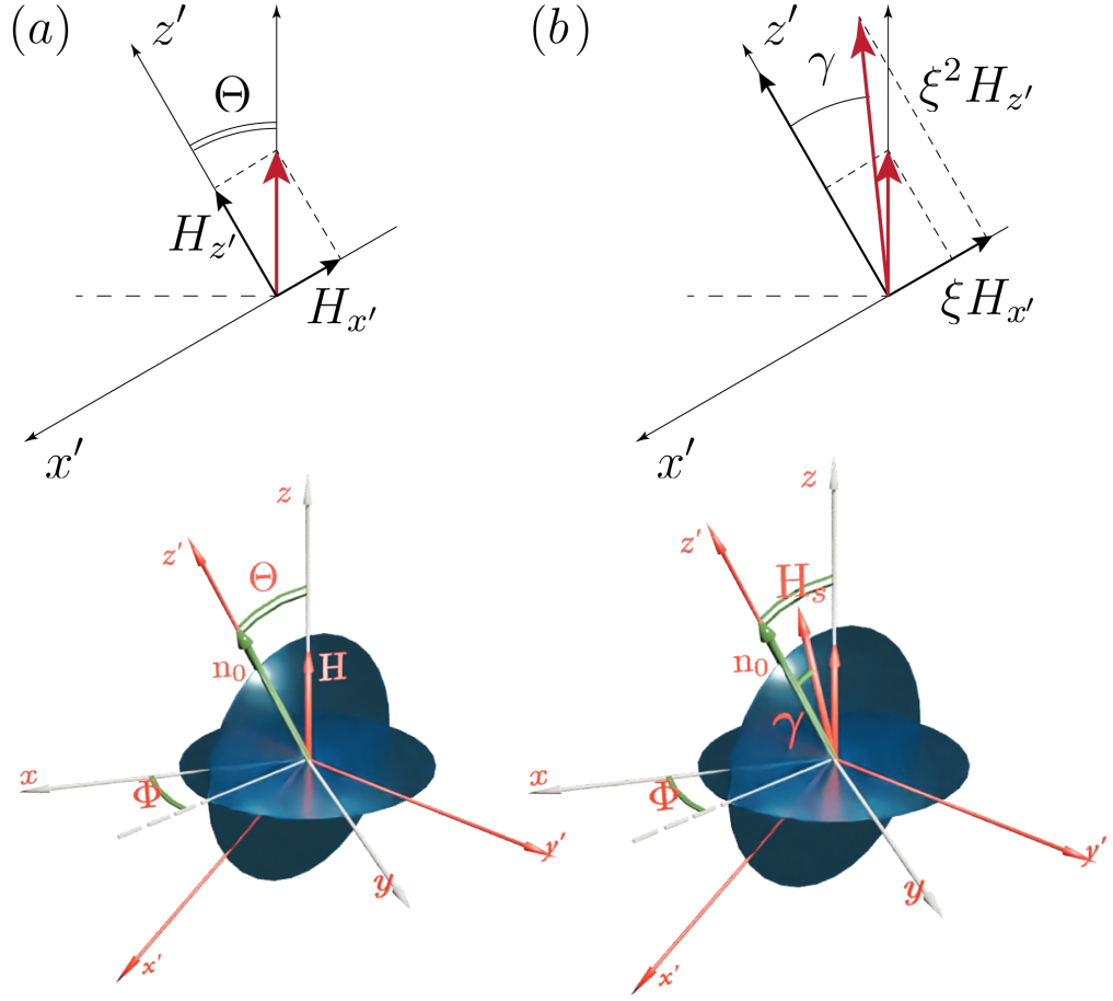
Рис. 2.2: (а) Повернутый базис x', y', z' . Ось z' ориентирована вдоль вектора анизотропии \mathbf{n}_0 . (б) Положение масштабированного вектора магнитного поля \mathbf{H}_s после масштабирования. Видно, что он остается в плоскости z'y' , но повернут на угол \gamma вокруг оси y' .
