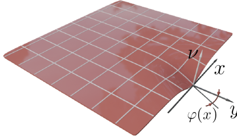
Рис. 3.1: Схематическая иллюстрация геометрического дефекта края в образце двумерного топологического изолятора
