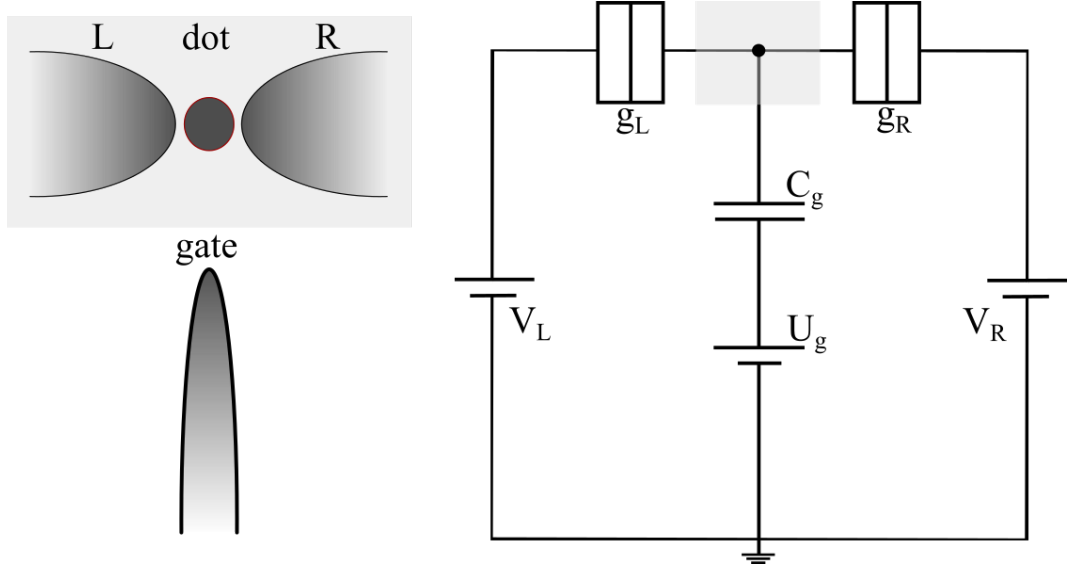
Рис. 1.1: Схематическое изображение одноэлектронного транзистора.
