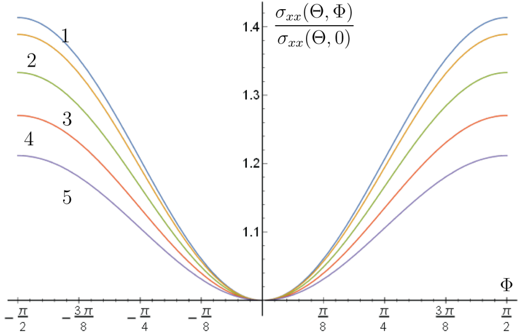
Рис. 2.4: Зависимость \Phi проводимости \sigma_{xx} при различных значениях полярного угла \Theta . Здесь \Theta уменьшается с шагом \pi/24 (см. кривые с 1 по 5); \Theta_n = \frac{\pi}{2} - (n-1)\frac{\pi}{24} . Графики построены при реалистичных значениях \xi = 4 ( \text{Cd}_2\text{As}_3 ) и постоянной тонкой структуры \alpha = 0,05 .
