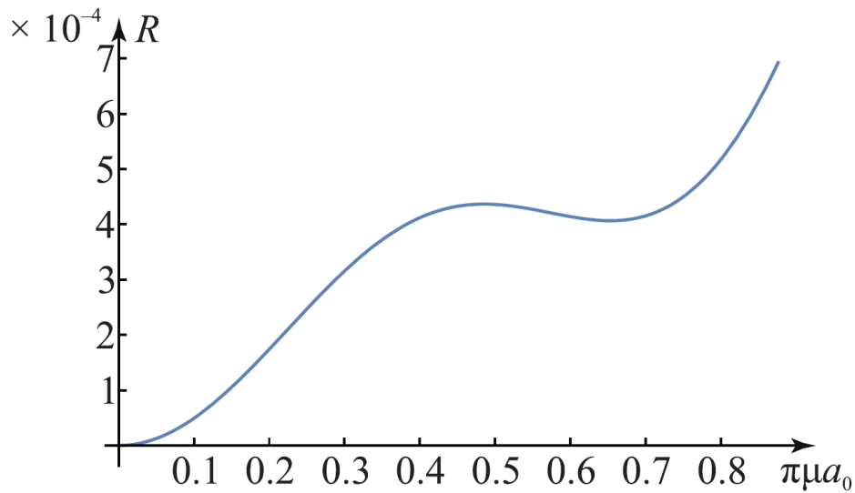
Рис. 3.7: Колебания коэффициента отражения (3.60), вычисленные для модельного потенциала \varphi(z) = (z - 8)e^{-z^2} , как функции параметра магнитного поля \pi\mu a_0 , где параметр a_0 \equiv |a|_{\mu=0} (см. (3.15)).
