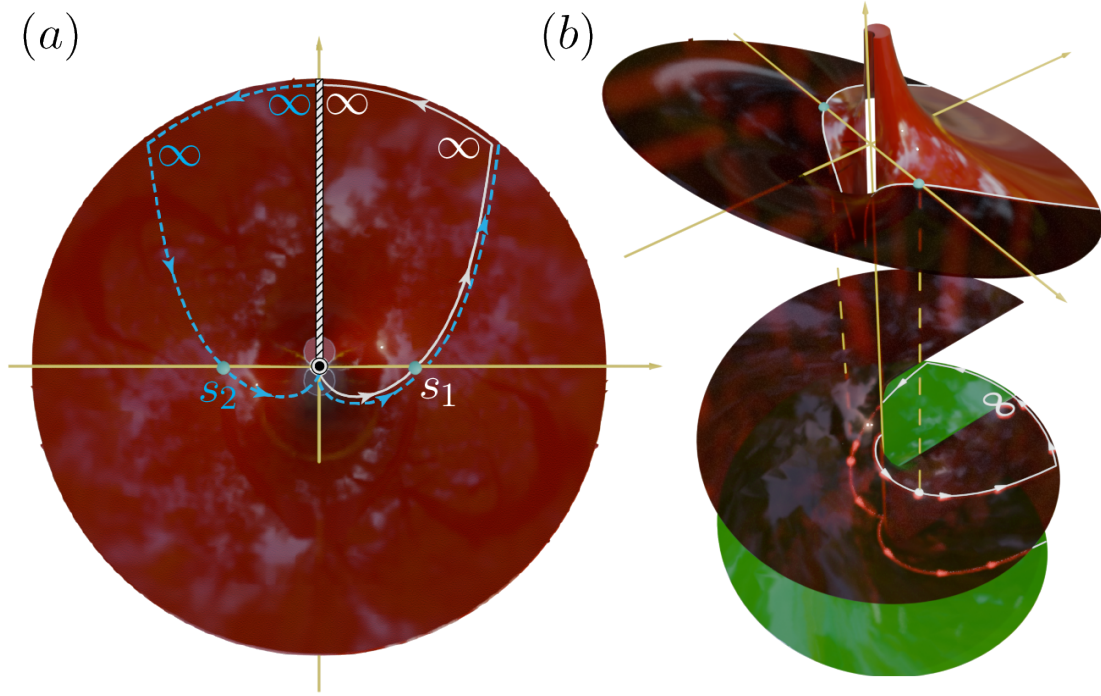
Рис. 3.6: (а) Контур наискорейшего спуска, дающий асимптотику точного решения (3.56) на левой антистоксовой линии. Голубой цвет означает размещение контура на другом римановом листе многозначной функции s^{ia\mu-1/2} из подынтегральной функции (3.56). (b) Вверх: Размещение контура на рельефе функции \text{Re}f(s, \zeta) . Вниз: Размещение контура на римановой поверхности функции s^{ia\mu-1/2} . Красный лист соответствует регулярной ветви s^{ia\mu-1/2} \equiv \exp((ia\mu - 1/2) \ln |s|) для s > 0 , а зеленый лист соответствует s^{ia\mu-1/2} \equiv \exp([ia\mu - 1/2][\ln |s| + 2\pi i]) для s > 0 .
