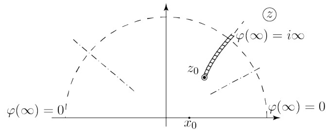
Рис. С.3: Схематическое поведение потенциальной функции \varphi(z) и \tau(z) . Пунктирные радианные линии обозначают границы изменения предела \varphi(\infty) .
