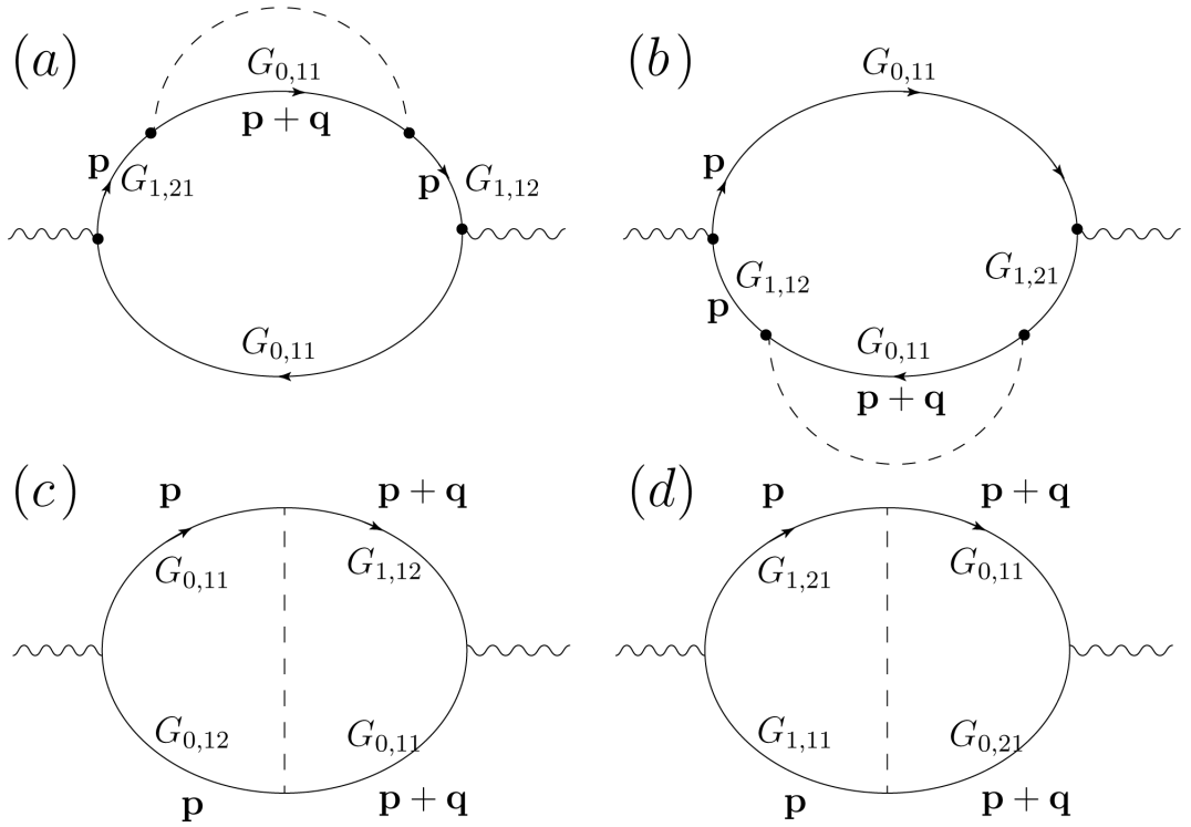
Рис. 2.3: Вклады первого порядка в проводимость \sigma_{xx} .
