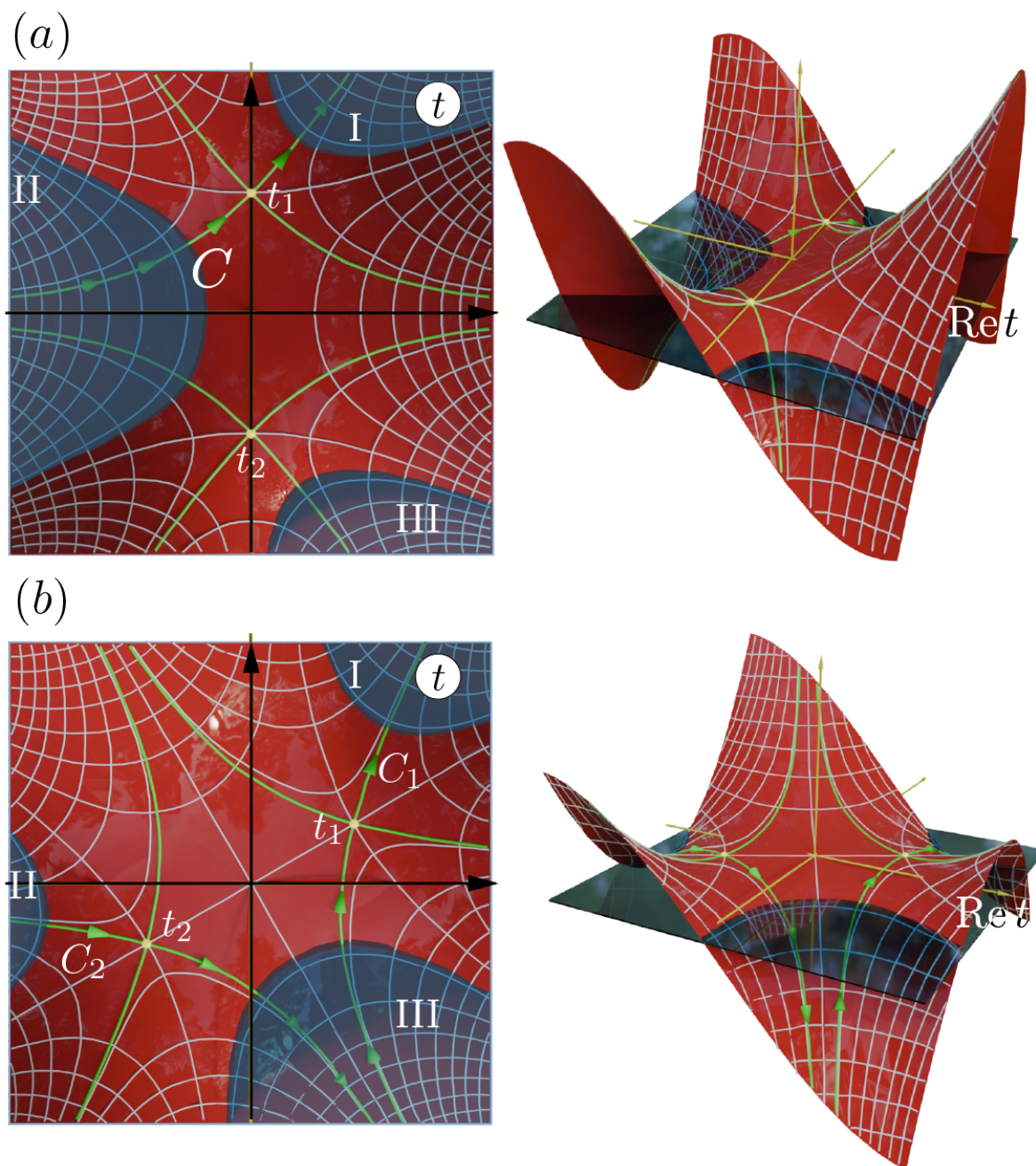
Рис. С.1: Рельеф действительной части функции f(t) = st + t^3/3 как функции t . Сетка состоит из стационарных линий f(t) . Тонкие зеленые контуры — это линии самого крутого спуска и подъема. Они пересекаются в двух седловых точках (маленькие желтые сферы). Мы также рисуем горизонтальную плоскость для наглядности. Плоскость очерчивает области (I, II, III), где значение \text{Re } f(t) стремится к -\infty . Это допустимые области для конечных точек размещения контура C (функция V(s) \rightarrow 0 в этих областях). Эти области также показаны серым цветом на рис. 3.3. (a) соответствует \arg s = 0 , (b) соответствует \arg s = -2\pi/3 .
