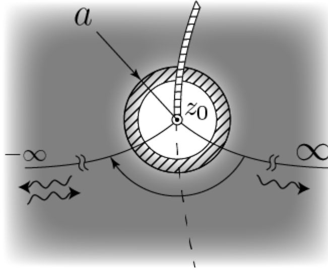
Рис. 3.2: К методу Покровского-Халатникова. Окрестность точки поворота z_0 со стандартным разрезом, идущим вверх. Серая область обозначает область применимости квазиклассического приближения (достигающую бесконечности в комплексной плоскости). Меньший круг радиуса a обозначает область применимости точного решения вблизи точки поворота. Две сплошные кривые, исходящие из точки поворота до \pm\infty , являются антистоксовыми линиями. Пунктирная линия — линия Стокса. Заштрихованная область — это область сосуществования квазиклассического и точного решения, в которых их можно сшить.
