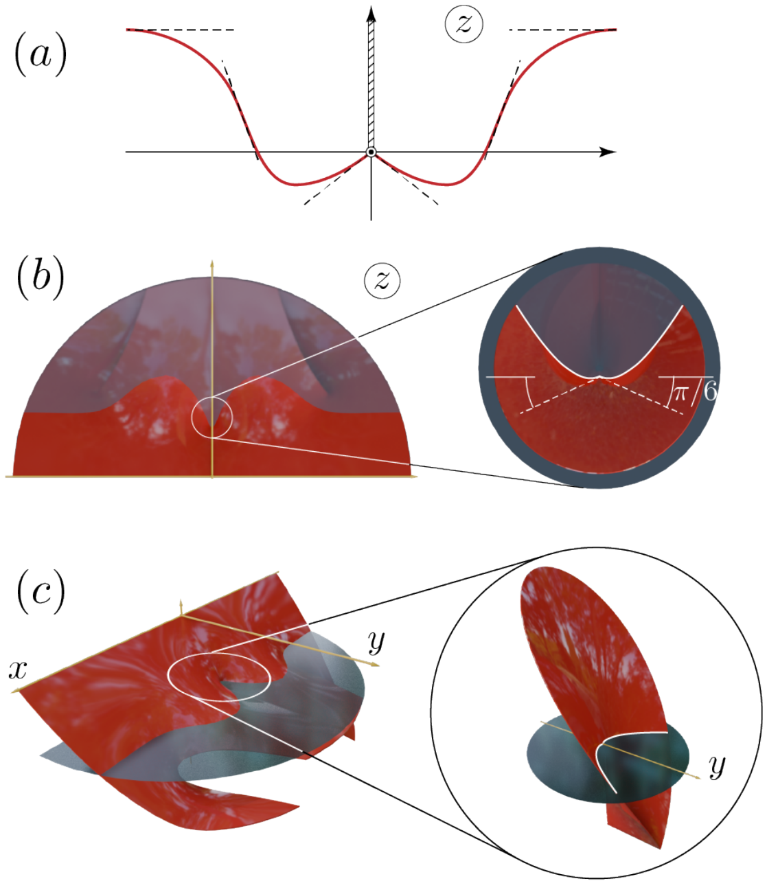
Рис. 3.4: (a) Структура антистоксовой линии из общих соображений. (b-c) Антистоксовы линии изображены как линии уровня функции i\text{Im} \int_0^\zeta \pi(t)dt с профильная функция \varphi(z) = ze^{-z^2/2} для \mu/\varepsilon = 0, 15 .
