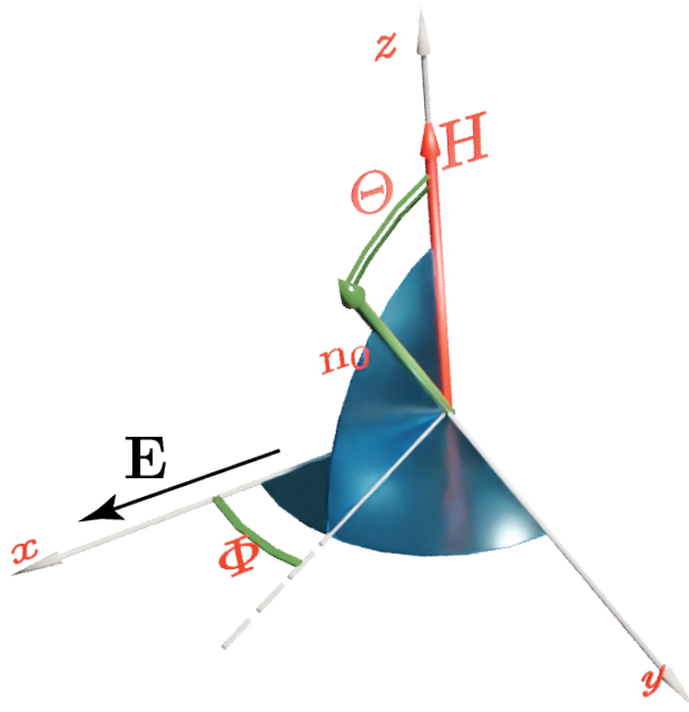
Рис. 2.1: Геометрия задачи. Ось анизотропии ( \mathbf{n}_0 ) наклонена на полярный угол \Theta и азимутальный угол \Phi . Напряжение приложено вдоль оси x .
